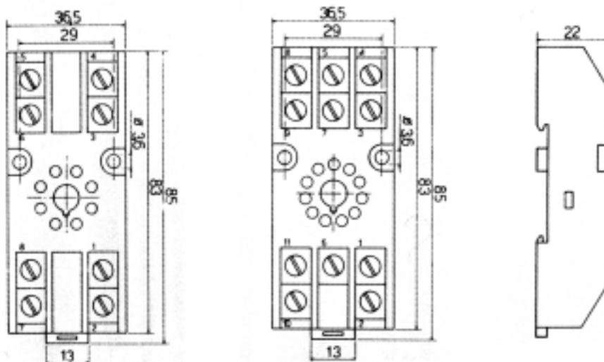
ZROV (8 pin)
