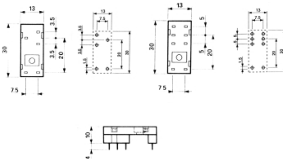
ZMECS/3 (for relays E31-F15A)
